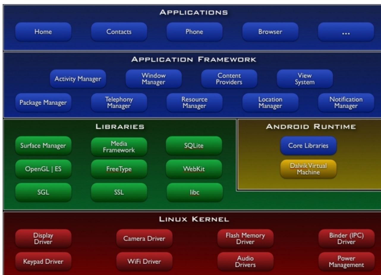
FIGURE 30.1. – L'architecture d'Android
