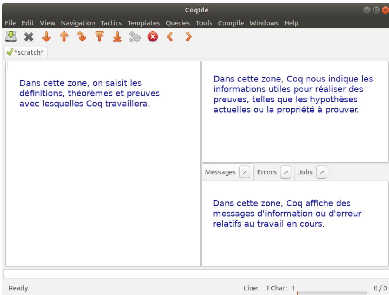
FIGURE 1.2. – L’interface de CoqIde.
