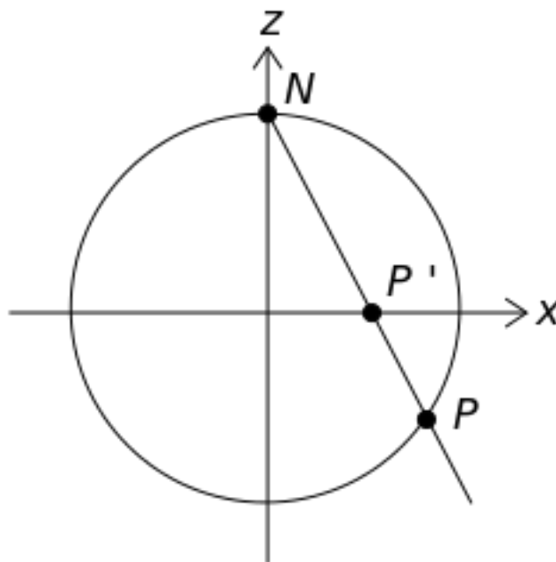
FIGURE 1.3. – Transformation birationnelle d’un cercle en droite par projection stéréographique ☞ (source ☞ ). Chaque point P du cercle est projeté sur un point P' de l’axe des abscisses.
